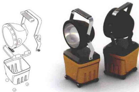
图1-8 应急灯设计: 邹玉清
