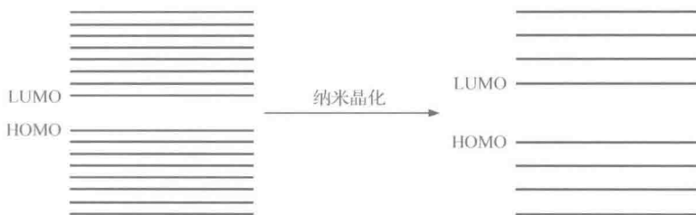
图 1.1 金属的量子尺寸效应示意图
