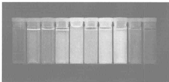
图 1-1 具有尺寸调制光发射性质的半导体量子点。本图所示为 ZnS 包覆的 CdSe 量子点,在近紫外灯的激发下,可以发射出从蓝色到红色的 10 种不同颜色的光,波长分别为 443 nm、473 nm、481 nm、500 nm、518 nm、543 nm、565 nm、587 nm、610 nm 和 655 nm [3]
