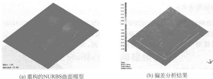
图 1-7 重构的 NURBS 曲面模型及其偏差分析
