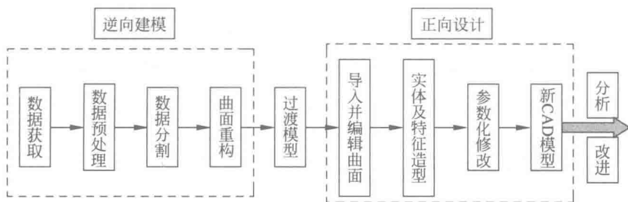
图 1-2 混合建模一般流程
