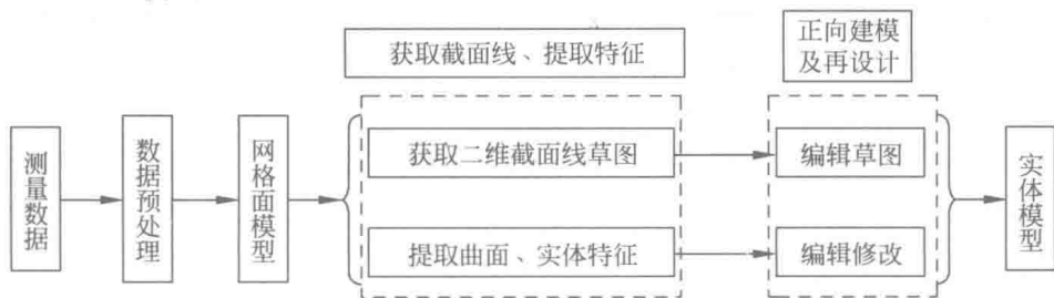
图 1-3 Geomagic Design Direct 混合建模流程
