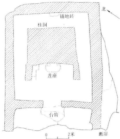
6. K18平面图
