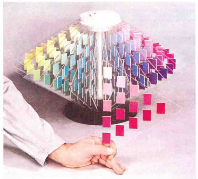
图 4-16 色立体图
