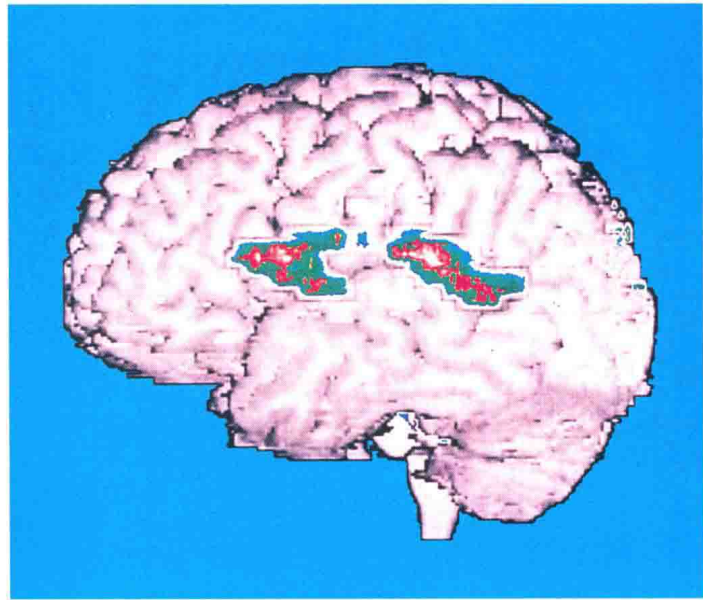
图 3-14 PET 扫描
