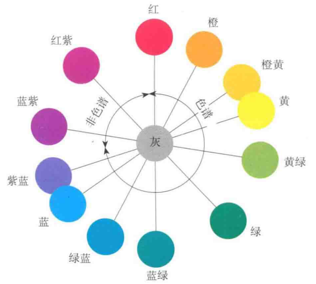
图 4-18 色环和补色
