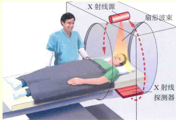
图 3-13 CT 技术
