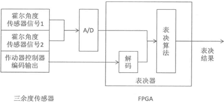
图 3 非相似三余度传感器系统方案
