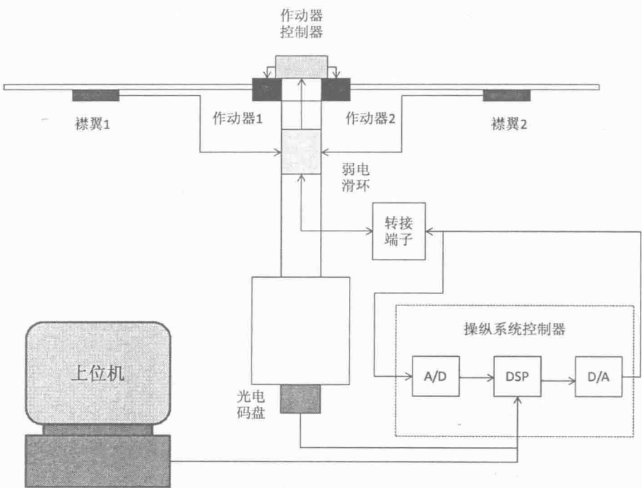
图 1 电控旋翼控制系统工作原理框图
