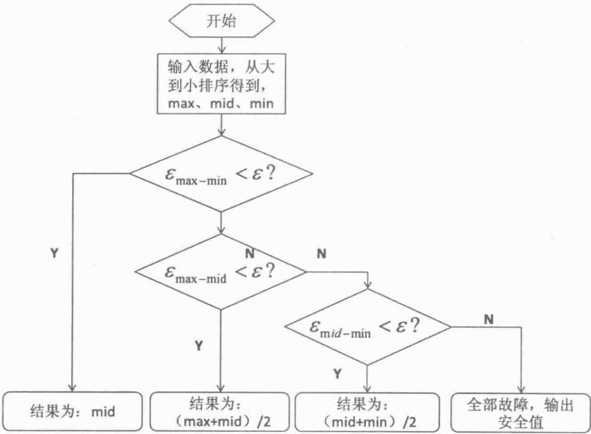
图 4 传统三余度表决策略的流程图
