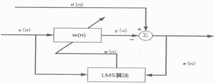
图 5 LMS 算法原理图
