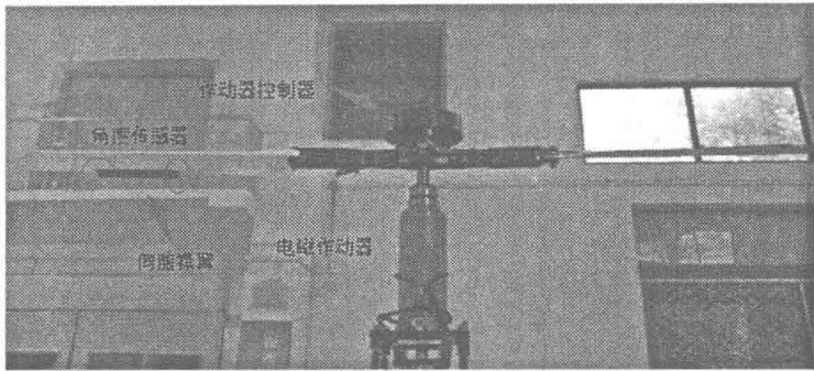
图 2 模型电控旋翼系统
