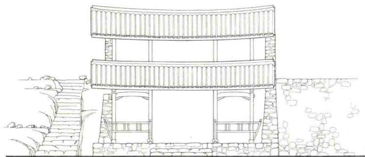
浙江永嘉楠溪江下垟头村路亭立面图
