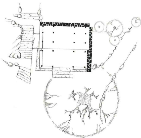
浙江永嘉楠溪江下垟头村路亭平面图
