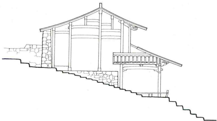
浙江永嘉楠溪江下烘头村路亭剖面图
