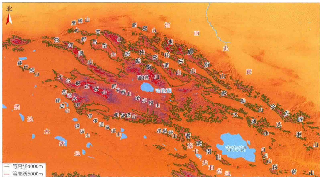
祁连山系组成示意图。祁连山地处青藏高原东北缘，由一系列大致平行的呈西北—东南走向的山脉和谷地组成，地势由东北向西南逐渐升高，海拔4000米以上的山地面积占整个山区面积的1/3以上。
