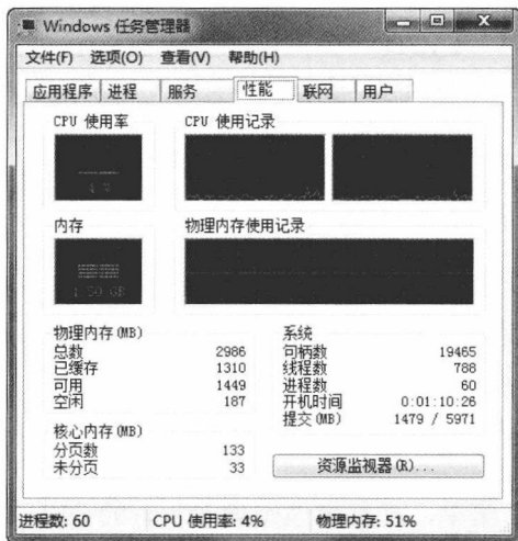
图 1-7 “性能”选项卡
