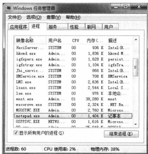
图 1-6 “进程”选项卡
