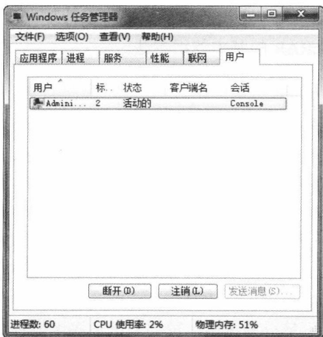
图 1-8 “用户”选项卡
