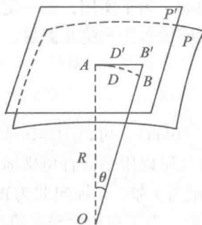
图 2-4 地球曲率对水平距离的影响
