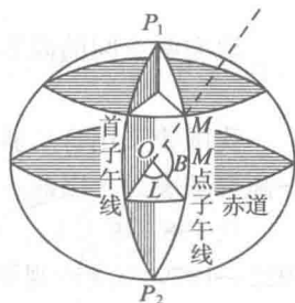
图2-2 地轴和两极
