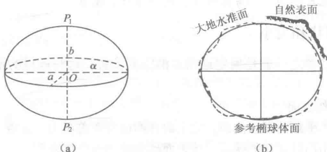
图 2-1 参考椭圆体
