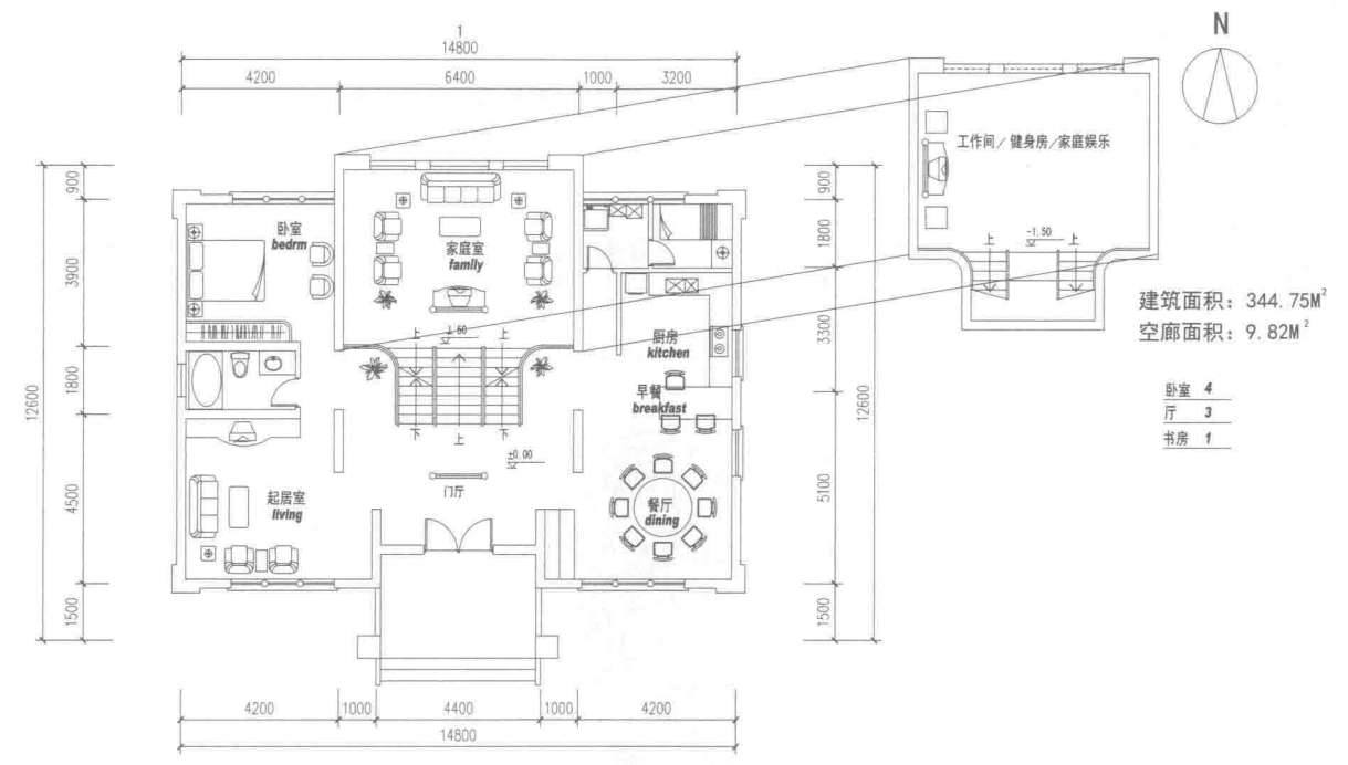
底层平面图
