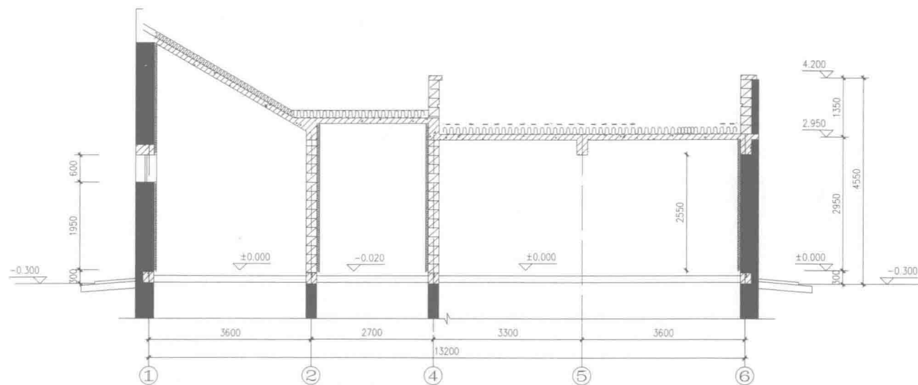
剖面图
