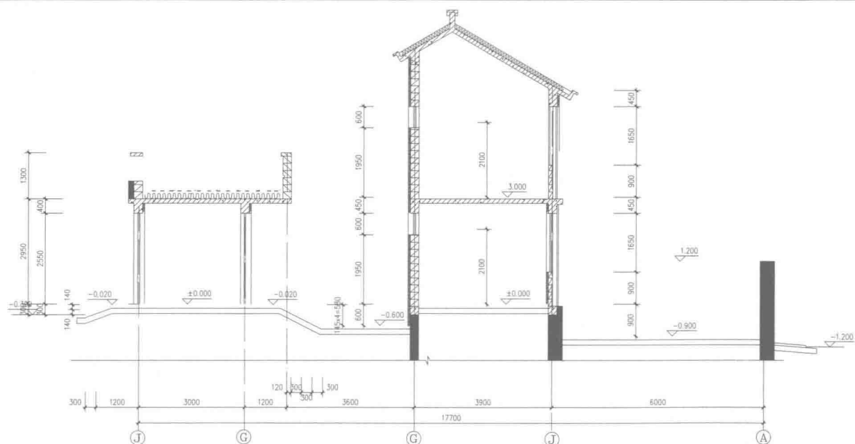
剖面图
