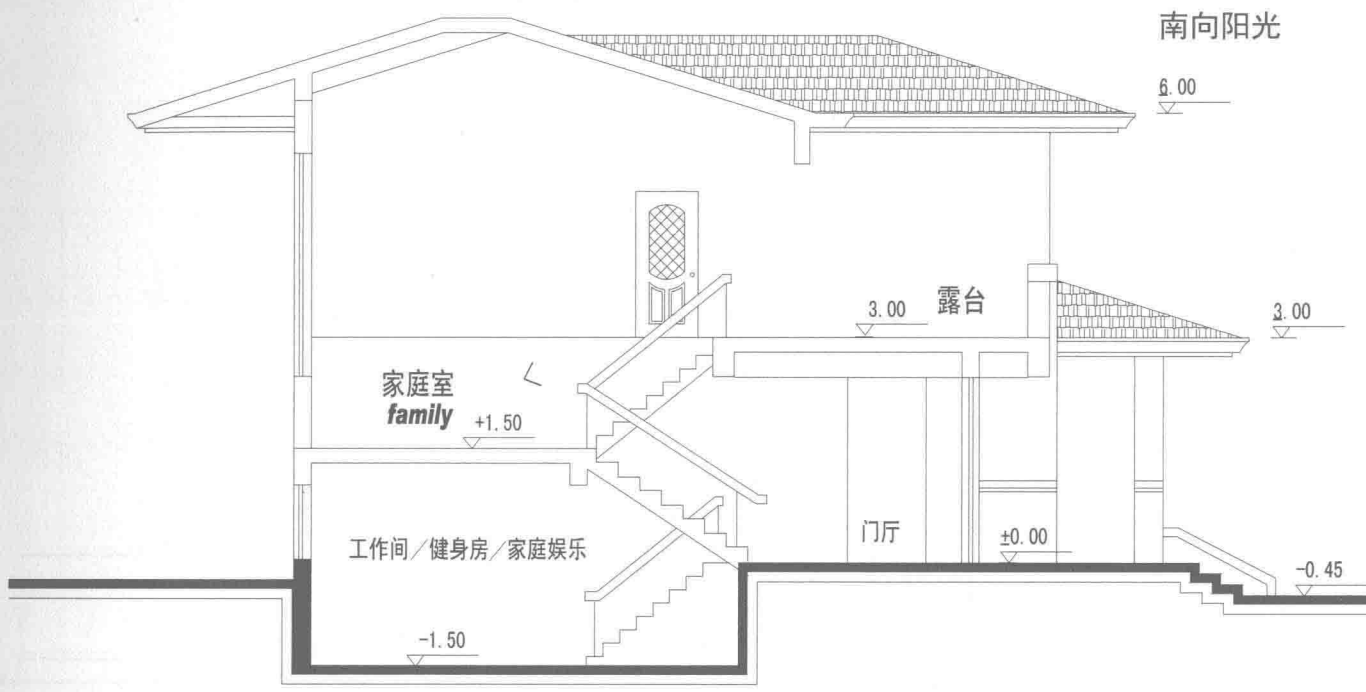
剖面图
