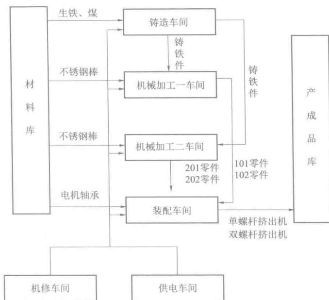
图 1-2 生产工艺流程
