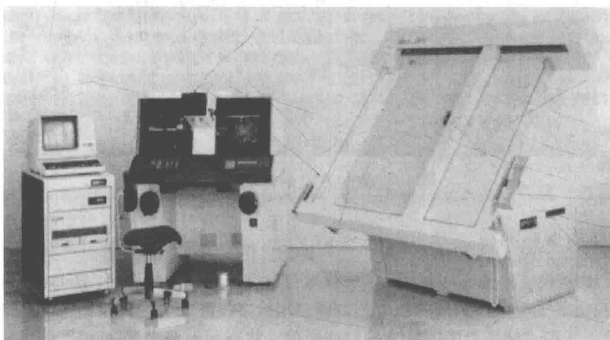
图 1.3 瑞士 Kern 厂 DSR-1 型解析测图仪
