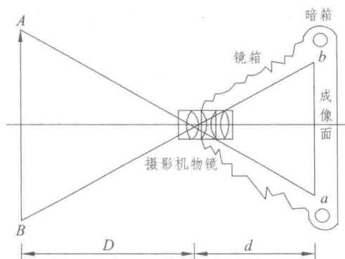
图 2.1 摄影机基本结构示意图
