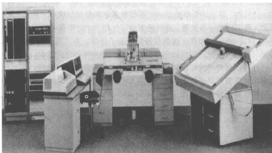
图 1.2 德国 Zeiss 厂 C-100 型解析测图仪
