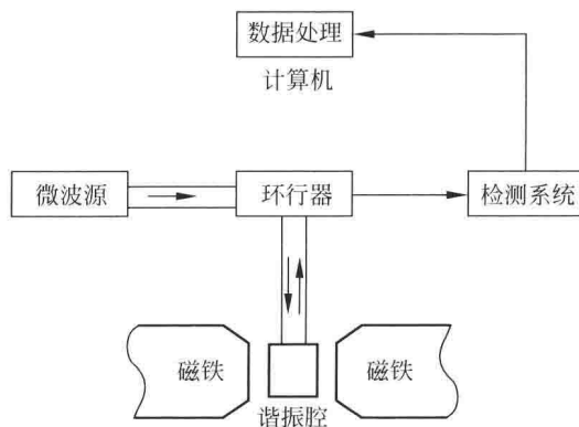
图 1.1 电子磁共振实验装置的原理框图
