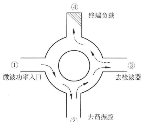
图 1.2 四端口微波环行器示意图
