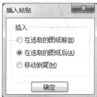
图 1-10 复制图纸
