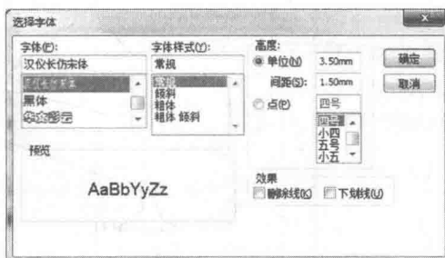
图 1-15 设置字体
