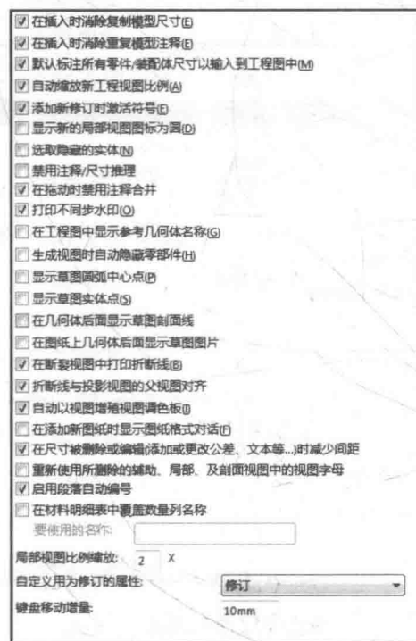
图 1-12 工程图选项
