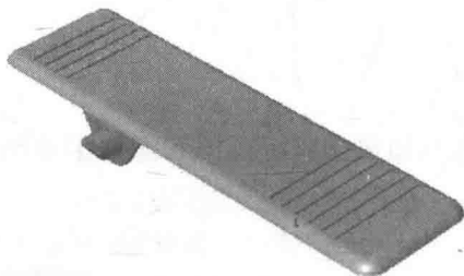
图 1-2 透视图
