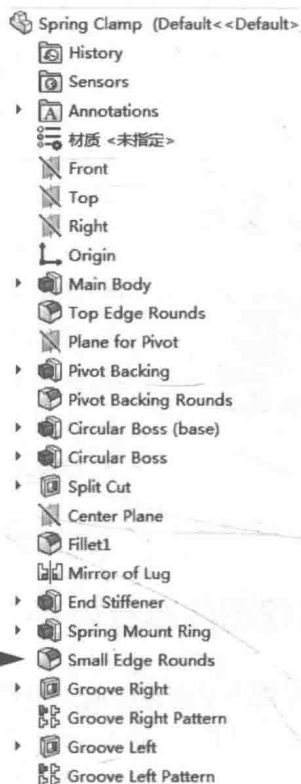
图 1-4 新配置 Simplified
