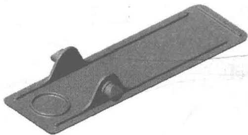
图 1-3 “反向” 视图
