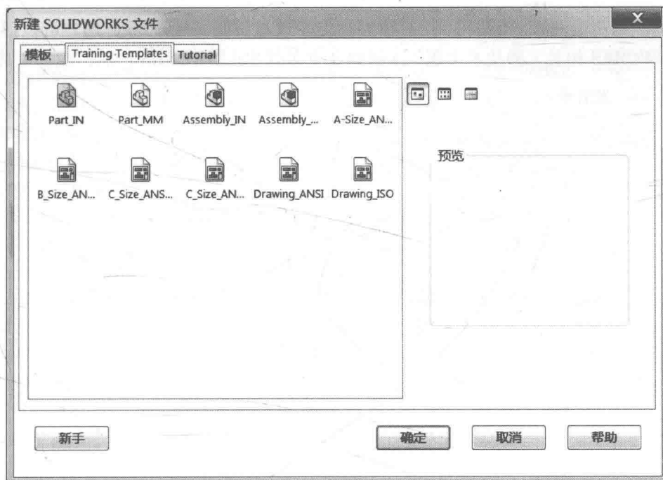
图 1 模板
