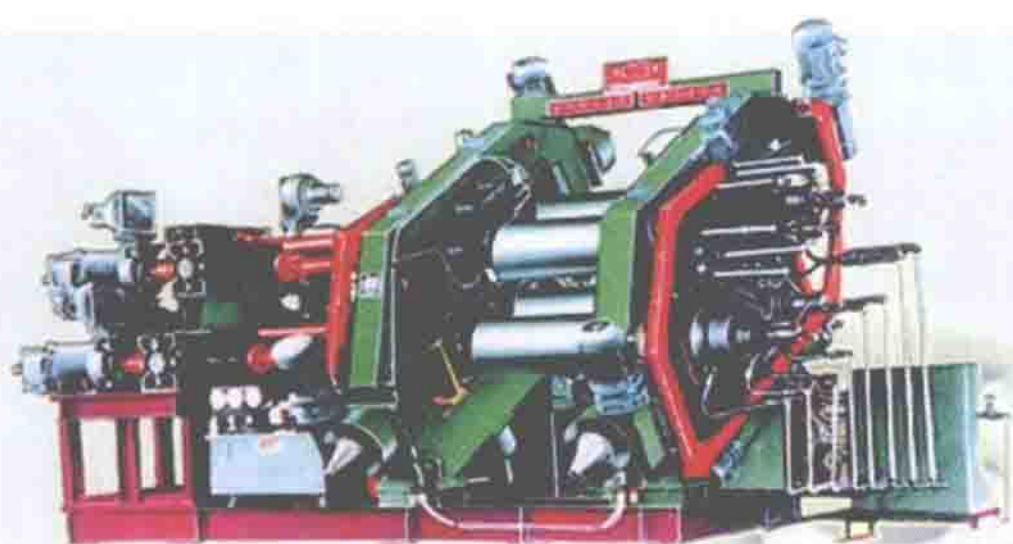
XY-4S 610 X 1730、XY-4S 400 X 1220 内衬层压延机
