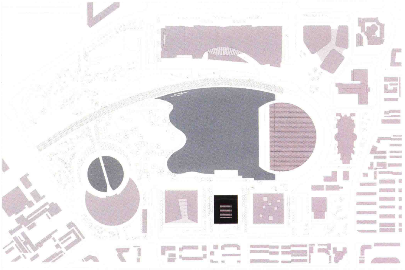
总平面图
