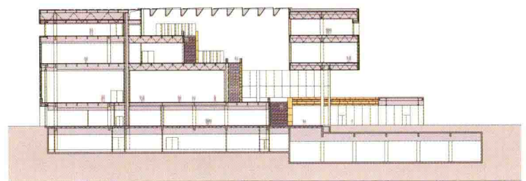
剖面图B-B
