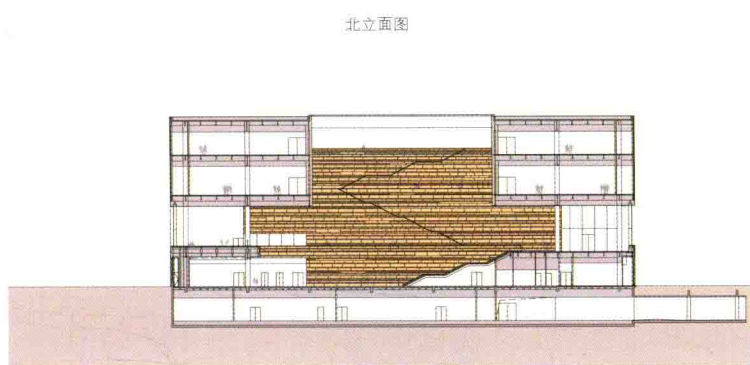
剖面图A-A
