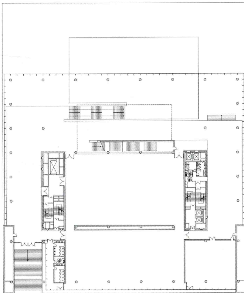
二层平面图
