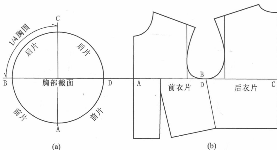
图 1-1-1 四开身结构
