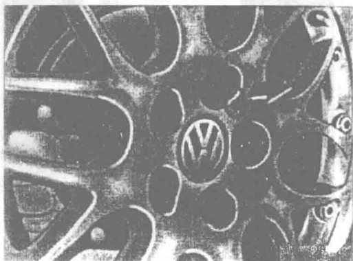
图 1-7 车轮螺栓防护帽的拆卸
