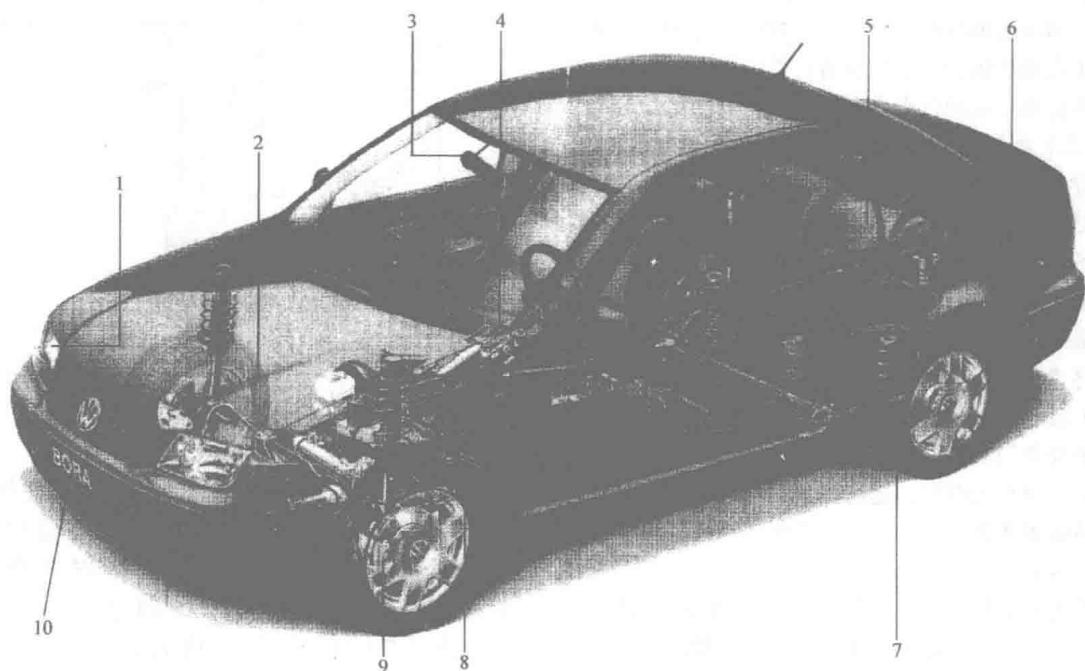
图 1-1 宝来轿车构造图
