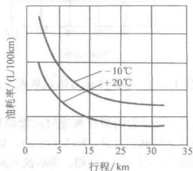
图 1-13 环境温度与油耗率的关系
