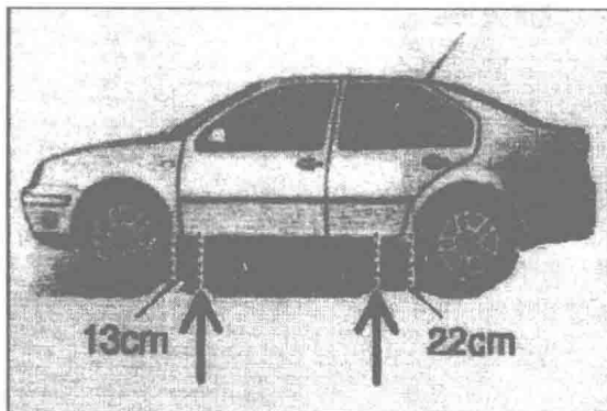
图 1-9 千斤顶安装位置
