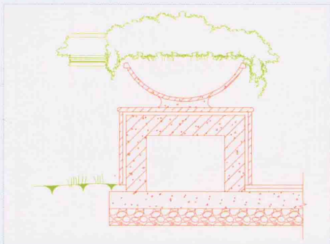
■ 花钵剖面图
