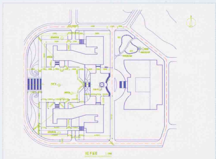
某校园B区平面图
