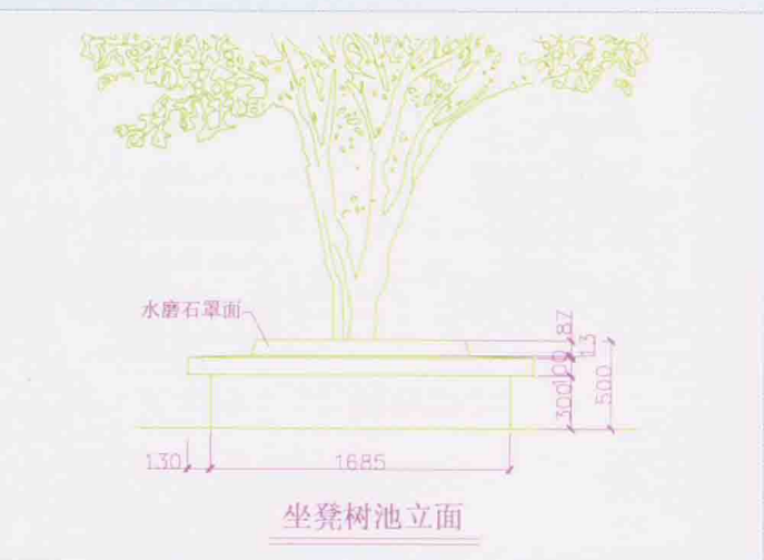
绘制坐凳树池立面图
