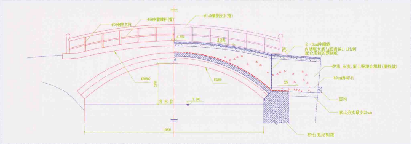
A-A剖面图
