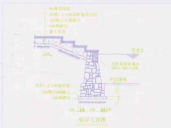
驳岸七详图
