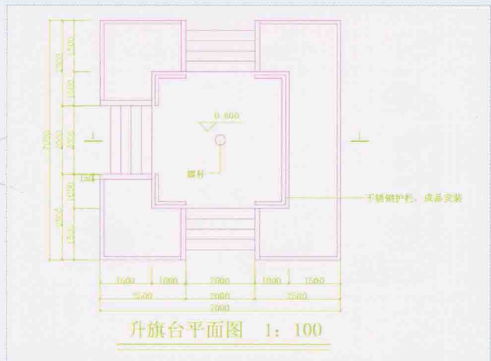
升旗台平面图
