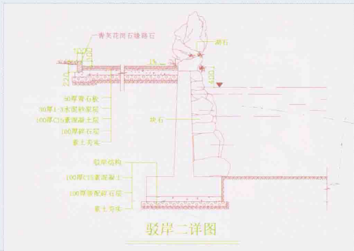
驳岸二详图
