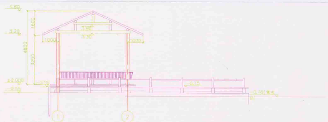
1-2 立面图
