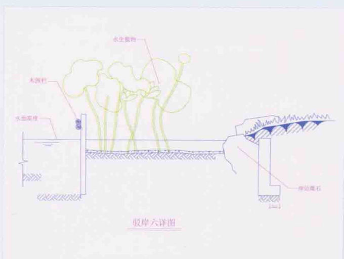
驳岸六详图
