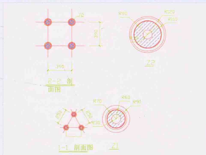
喷泉详图
