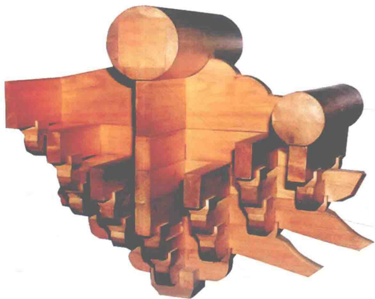
斗拱(模型)
