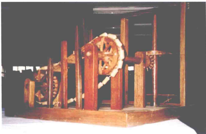
高筒转车(模型)
