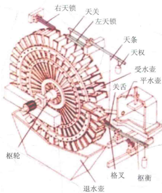
水运仪象台擒纵装置
