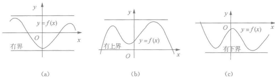
图 1-7 函数的有界性
