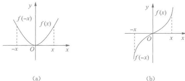
图 1-8 函数的奇偶性
