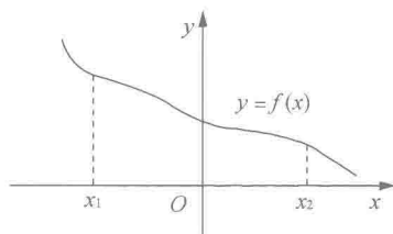
图 1-5 单调减少函数图像
