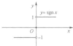
图 1-2 y=\operatorname{sgn} x 的图像
