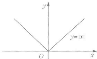
图 1-1 y=|x| 的图像
