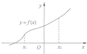
图 1-4 单调增加函数图像
