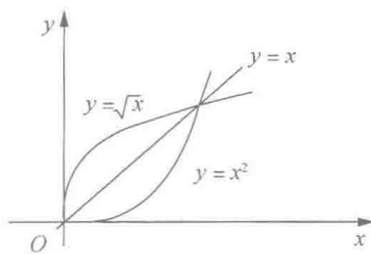
图 1-9 y=x^2 与 y=\sqrt{x} 的图像
