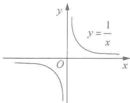
图 1-6 y=\frac{1}{x} 的图像
