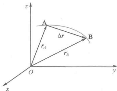
图 1-2 质点的位移
