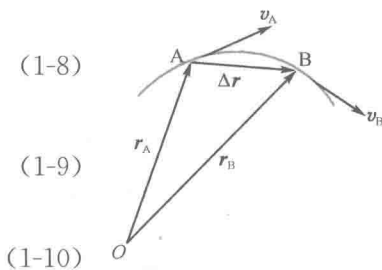
图 1-3 质点的速度
