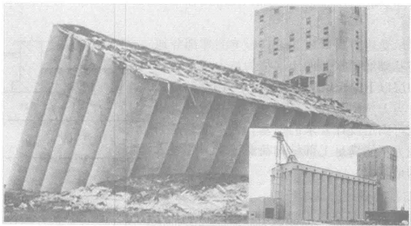
图 0-2 加拿大 Transcona 谷仓
