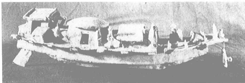
插图 13. 公元 1 世纪的广州墓穴出土的汉代陶船模型;这是所有文化中已知最早的艏柱舵例证。
