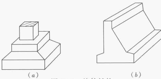
图 10-3 块体结构
