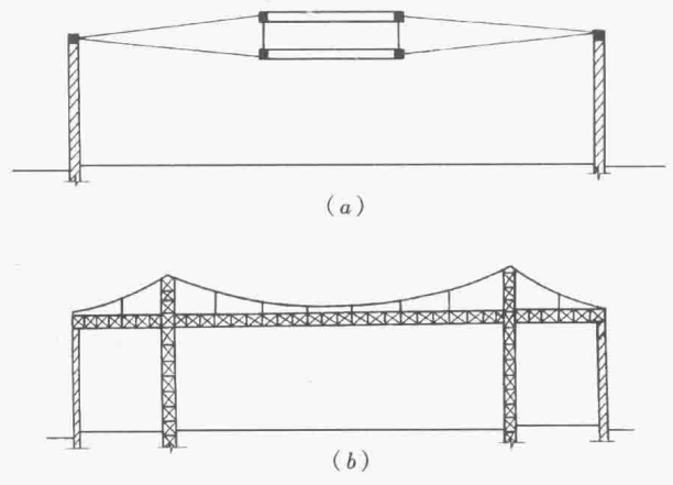
图 10-4 索结构
