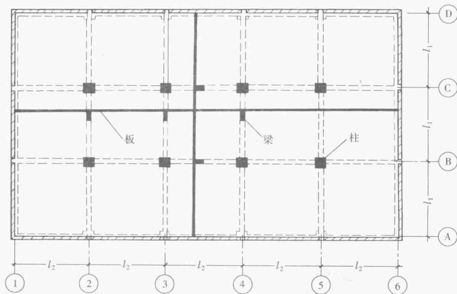
图 11-2 双向板肋形楼盖
