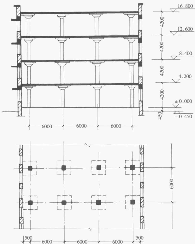
图 11-4 无梁楼盖
