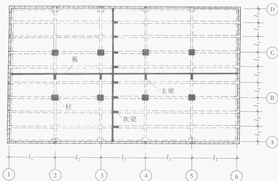
图 11-1 单向板肋形楼盖
