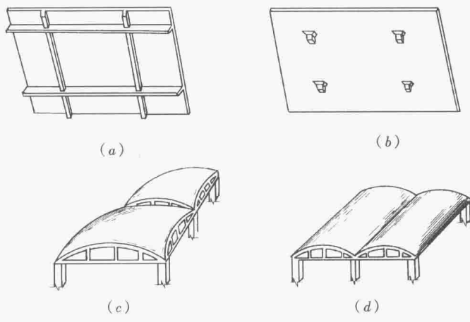
图 10-2 板和壳结构
