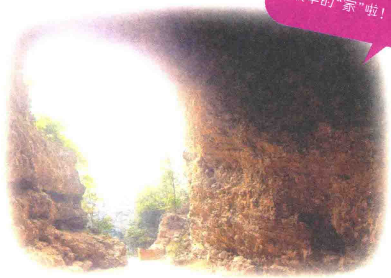
图 1.2.1 猿人洞
