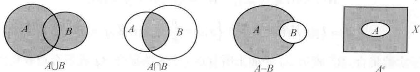
图 1.1 集合的四种运算图示
