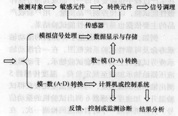
图 0-1 测试系统的一般组成
