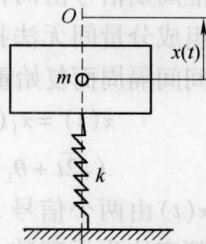
图 1-1 单自由度振动系统
