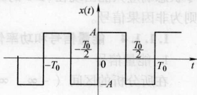
图 1-8 周期方波
