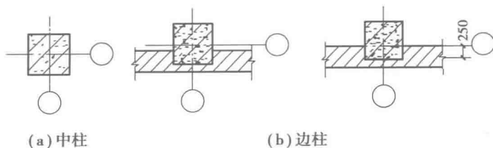
图 1.8 框架结构柱定位轴线
