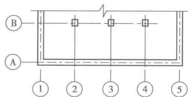
图1.3 定位轴线的编号顺序
