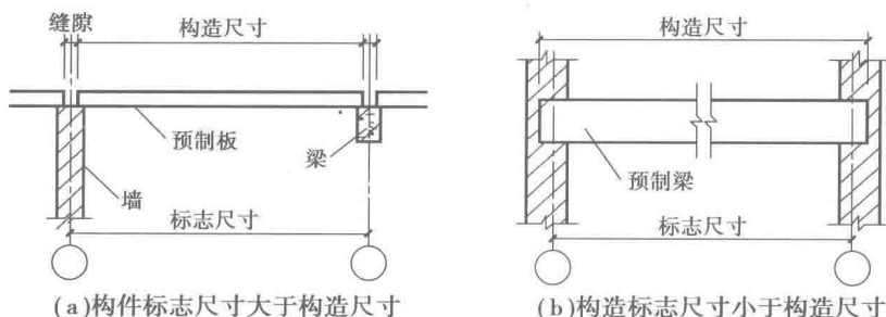
图1.2 几种尺寸间的关系
