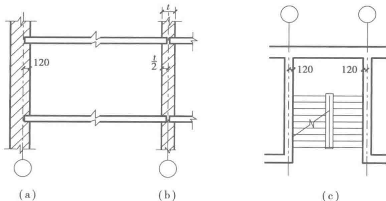
图 1.7 混合结构墙体定位轴线
