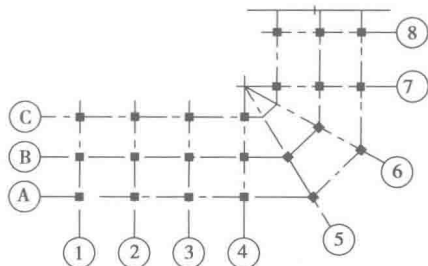
图 1.6 折线形平面定位轴线的编号
