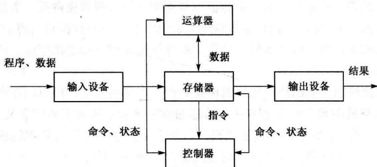
图 1-1 计算机组成示意
