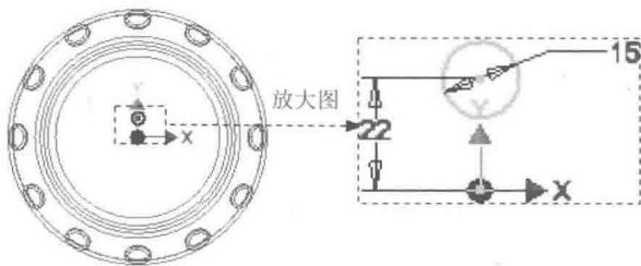
图 1.17 截图草图
