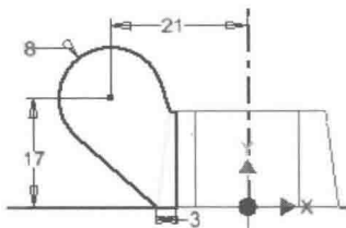
图 2.5 截面草图
