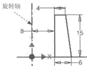
图 2.3 截面草图
