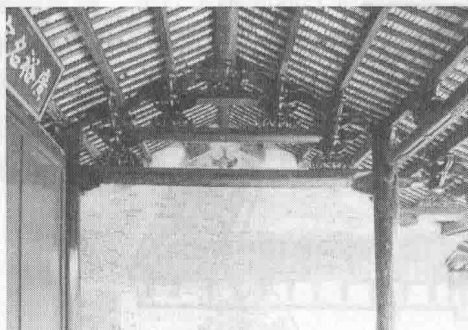
图 1-6 抬梁(叠架)式
