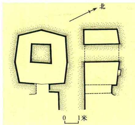
克孜尔尕哈第24窟平、剖面图
