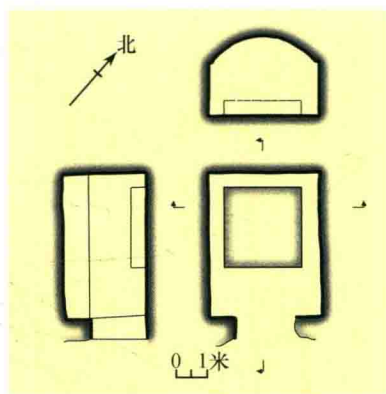
阿艾石窟平、剖、立面图
