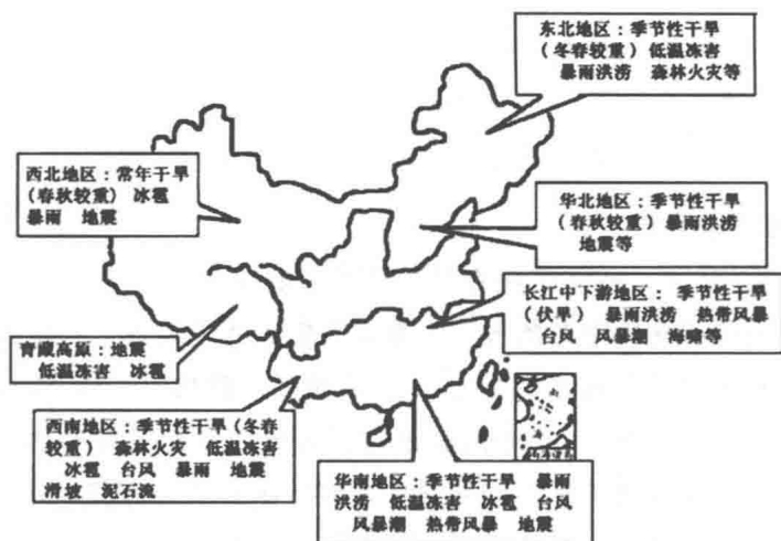
图 0-1 中国自然灾害分布地域
