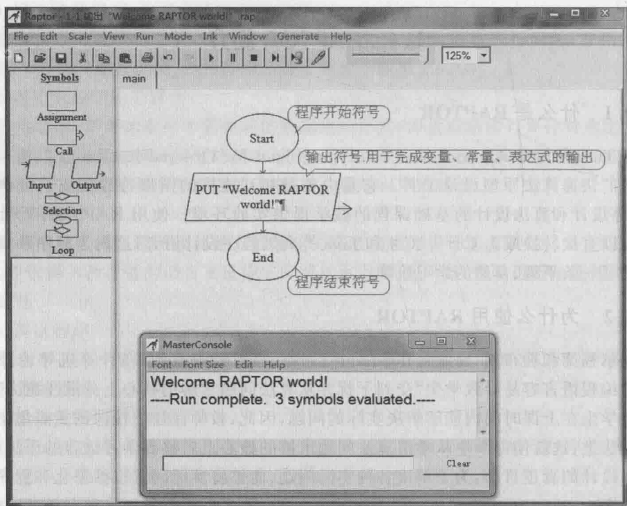
图 1-3 简单 RAPTOR 程序设计及运行结果
