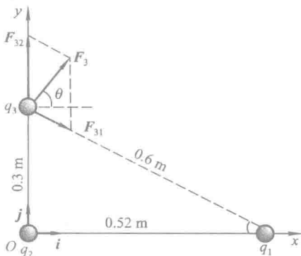
图 10-2 求作用在 q_3 上的合力
