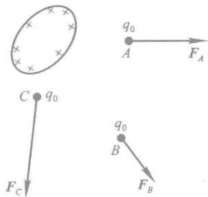
图 10-3 试探电荷 q_0 在电场中受力的情况
