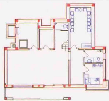
地下室装饰平面图
