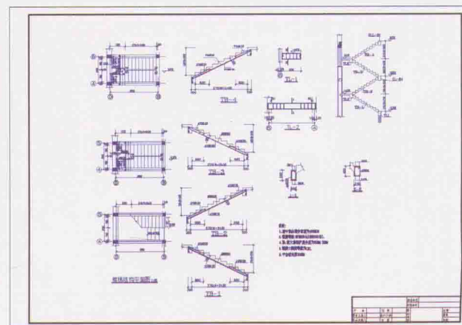
楼梯结构配筋图
