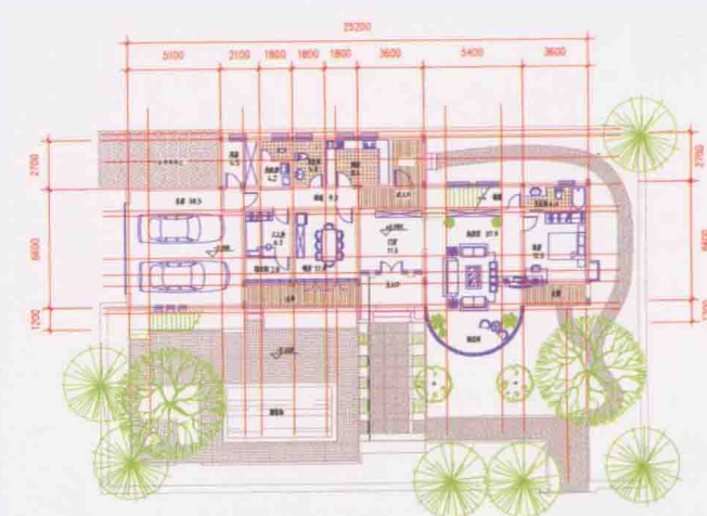
■ 底层平面图
