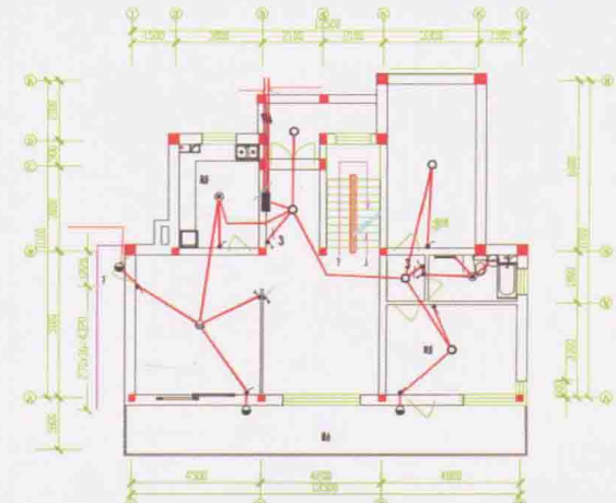
■ 首层照明平面图的绘制
