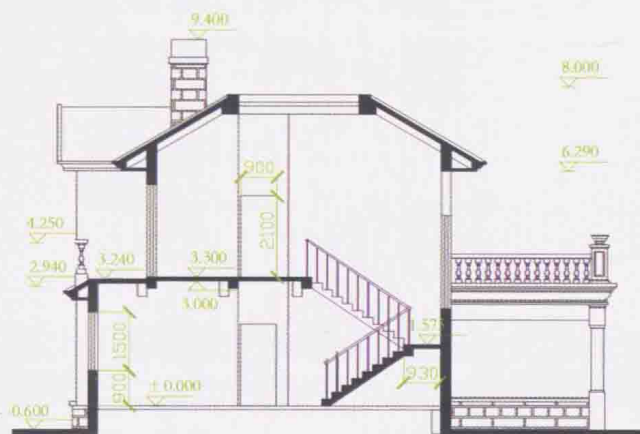
别墅1-1剖面图
