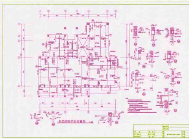
首层结构平面布置图
