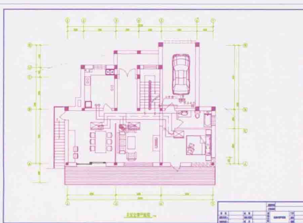
首层空调平面图
