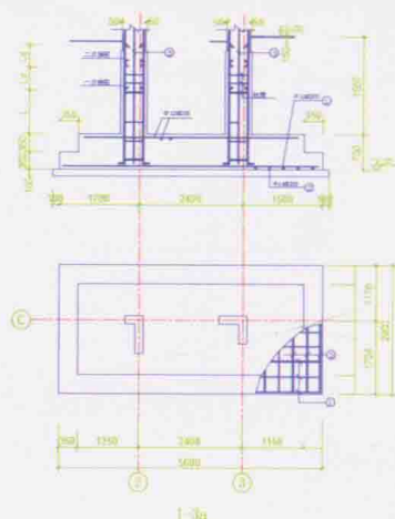
■ 别墅结构基础大样详图二
