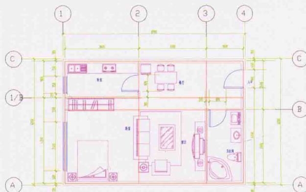
居室室内设计平面图 1:50
