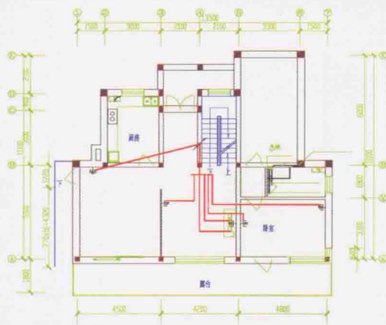
■ 首层电视电话平面图
