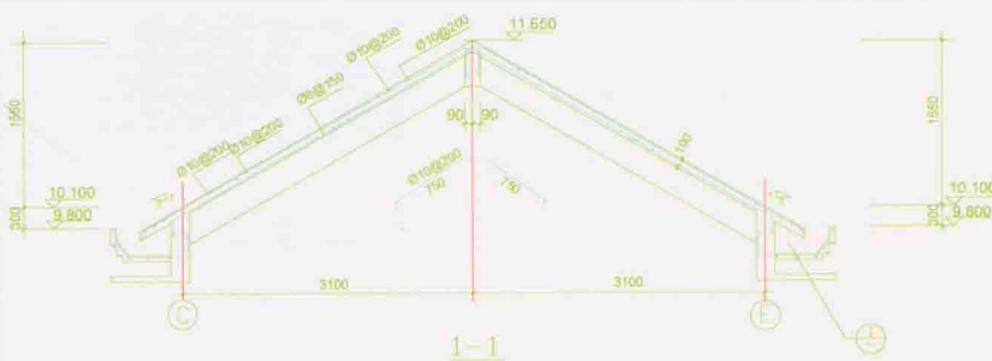
1-1剖面配筋图
