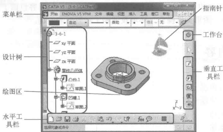
图 1-3 软件界面
