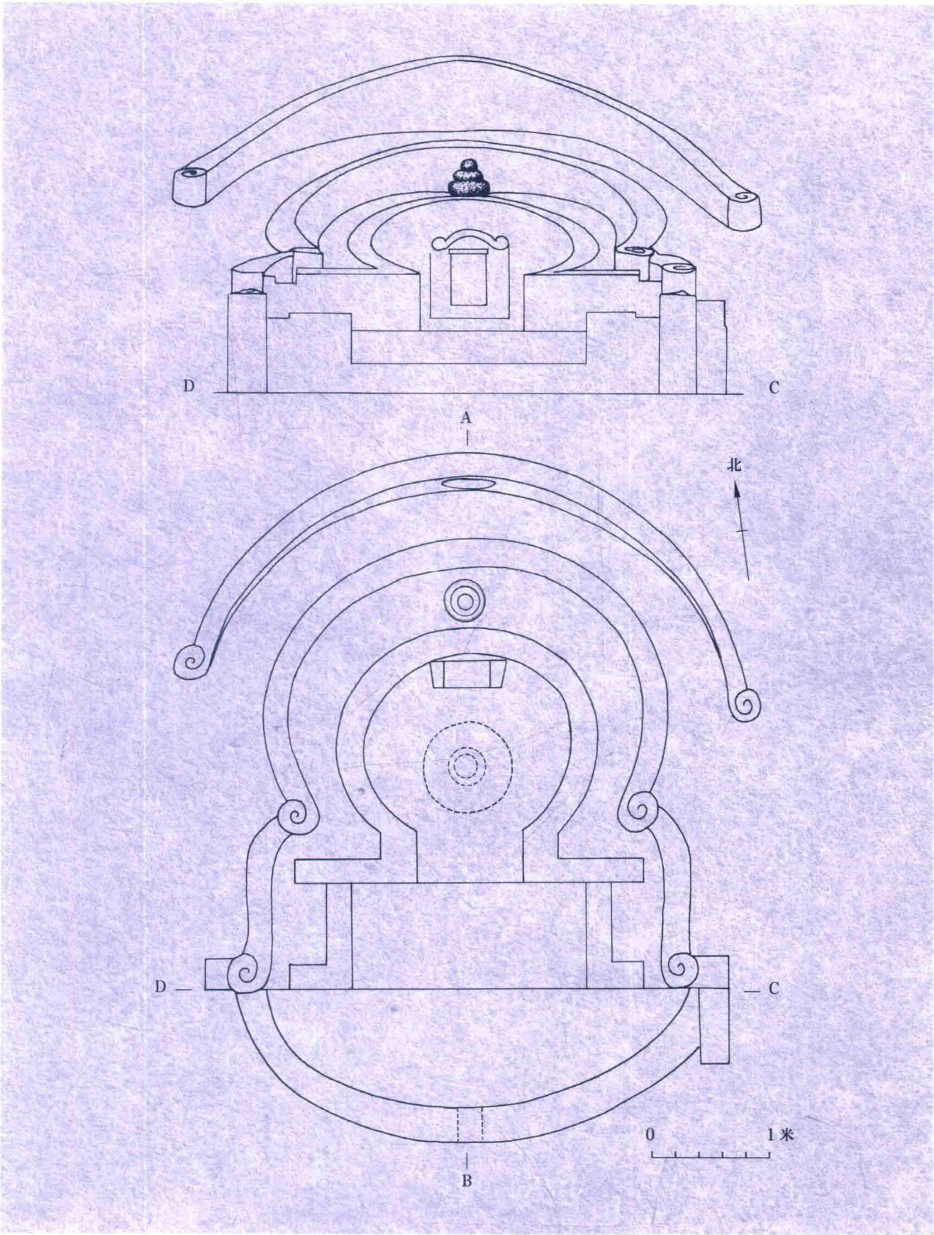
图四 M1 平、立面图
