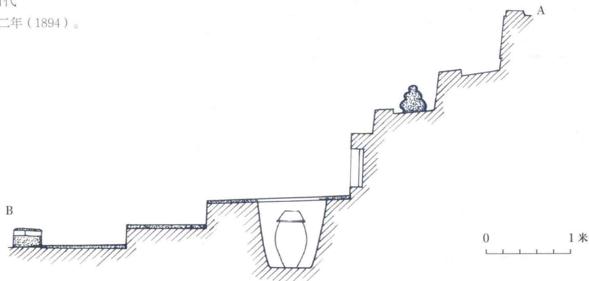
图三 M1 剖面图
