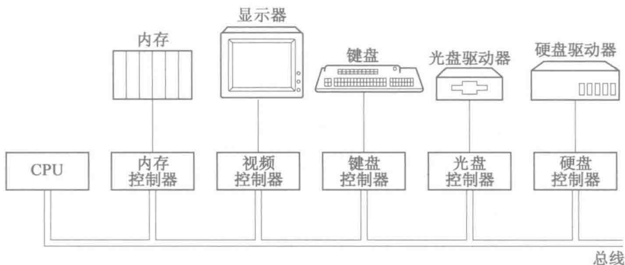
图 1-1 现代计算机系统的硬件结构
