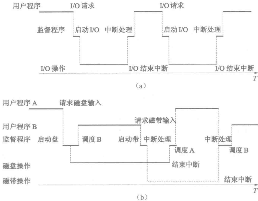
图 1-2 单道程序和两道程序的运行情况
