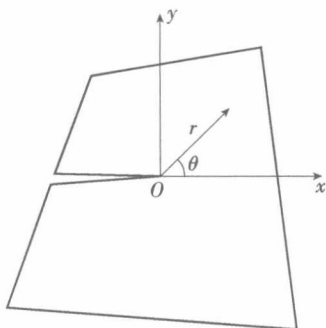
图 2.1 含边缘裂纹的二维固体
