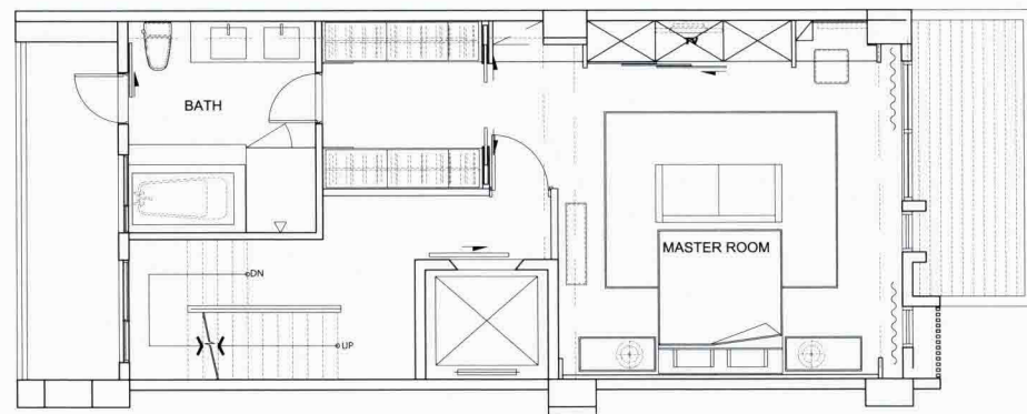
三层平面图
