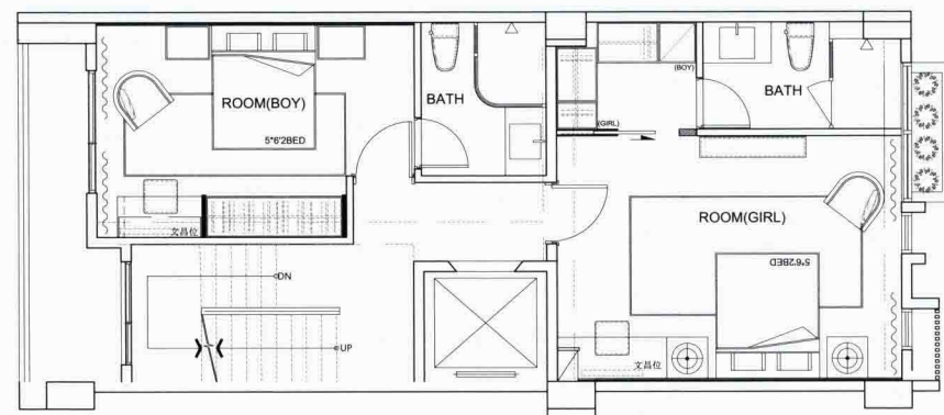
四层平面图
