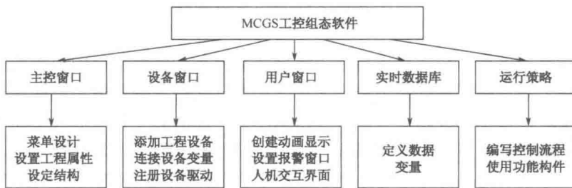
图 1-1 组态环境结构示意图
