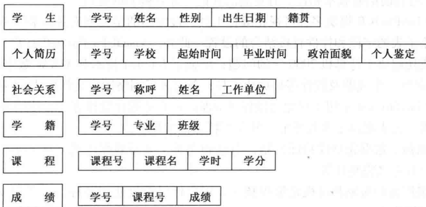
(c) 关系模型
