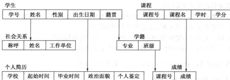
(b) 网状模型
