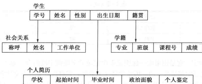
(a) 层次模型
