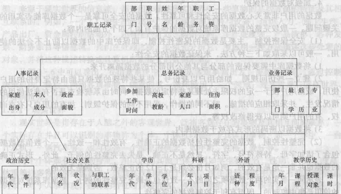
图 1-8 组合后的数据结构
