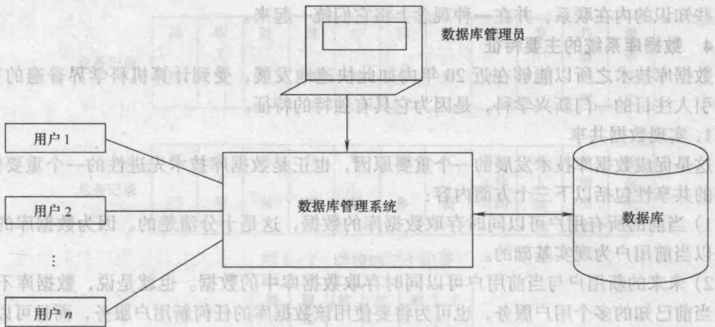
图 1-5 数据库系统
