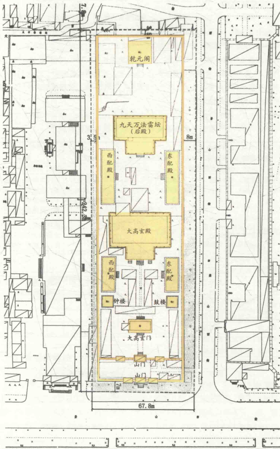
图五 大高玄殿现状实测图
