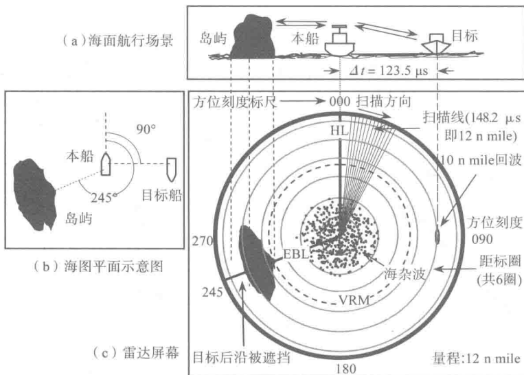
图2-1-1 雷达图像
