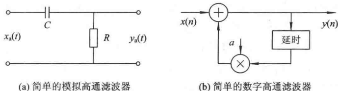
图 0.0.1 高通滤波器简型
